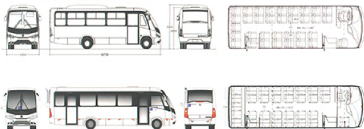
Carrocería con chasis Mercedes Benz LO-916
